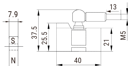
Магнит-ползунок (слайдерный магнит) Код заказа: « ПМ »
